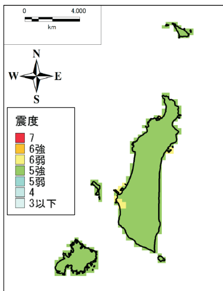
【震度分布】
