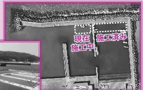
型枠ブロック設置完了写真
