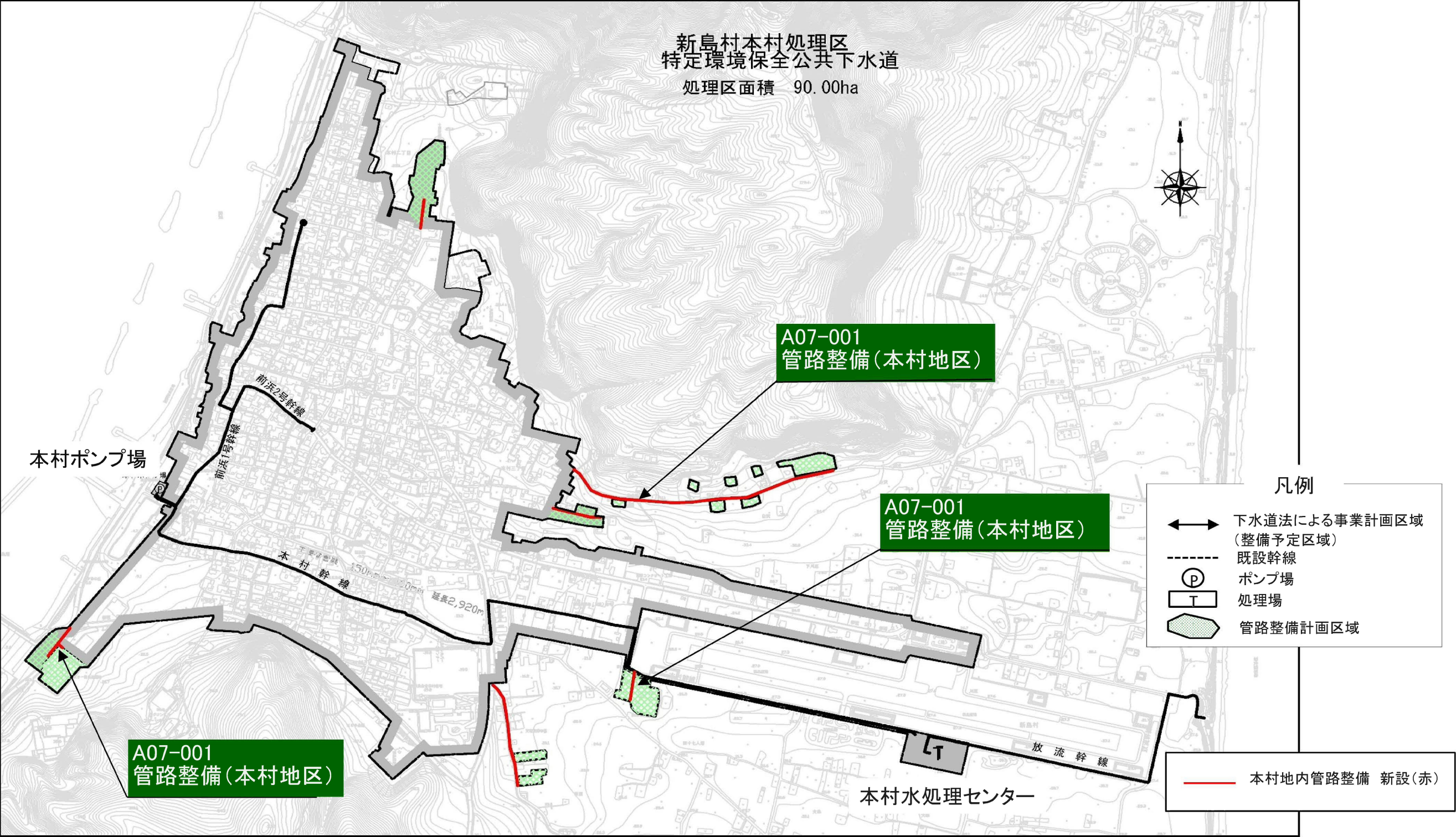
本村処理区計画図
